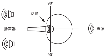
握持示意
